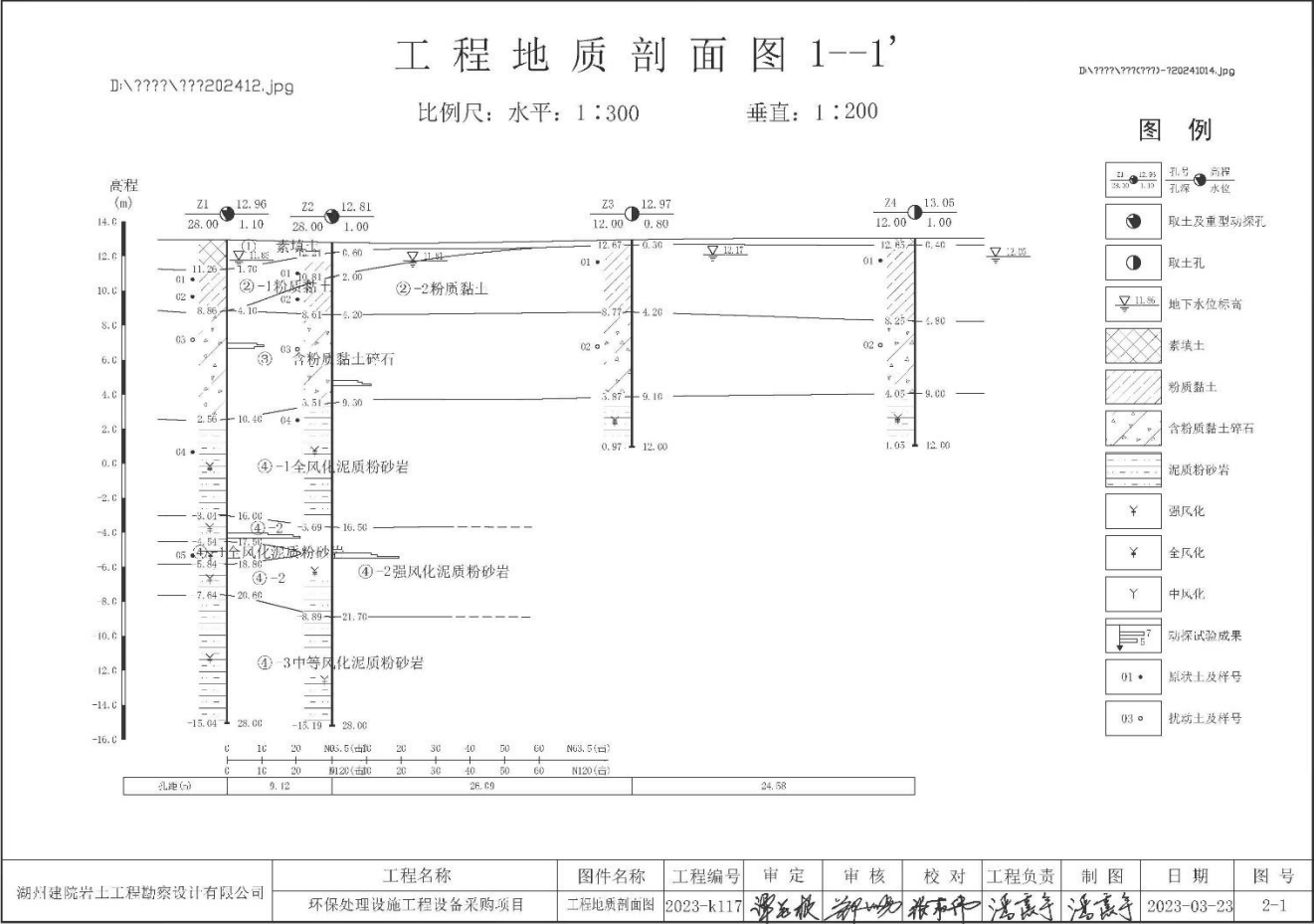
图 3.1-5 地质剖面图（2023 年）
