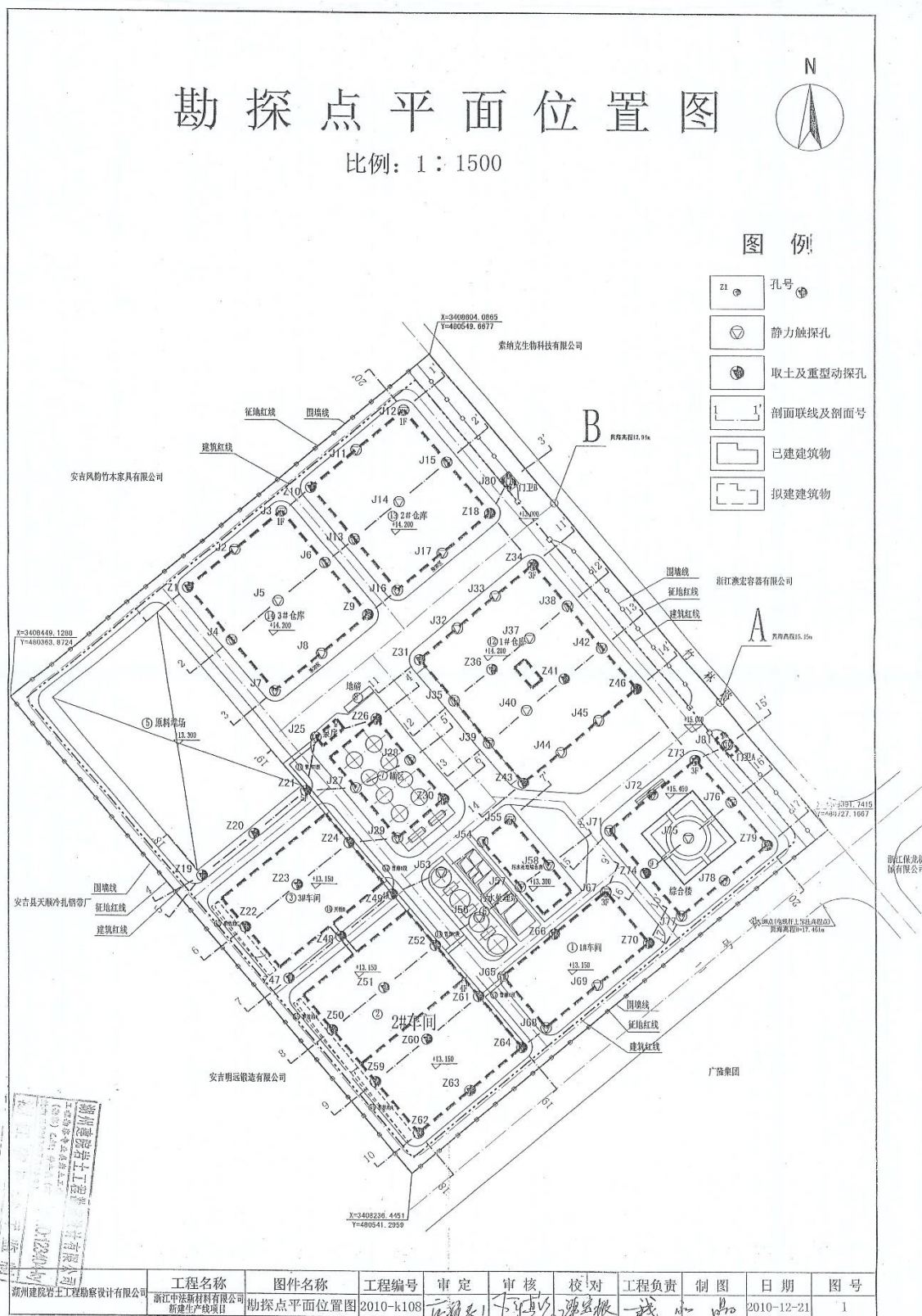
图 3.1-2 勘探平面图 (2010 年) 16
