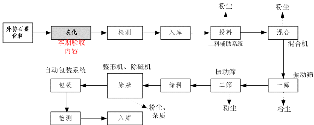
图 2-7 实际工艺流程及产污环节图
