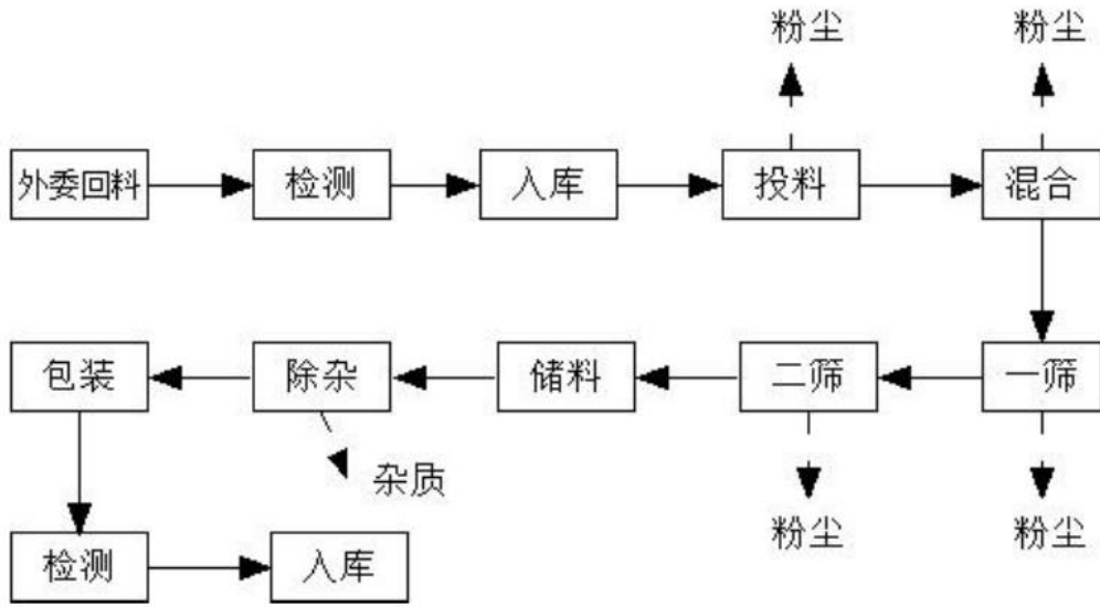
图 2-7 后端环节工艺流程及产污环节图（环评描述）
