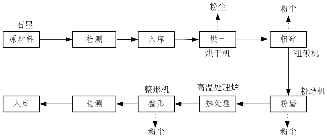
前端环节生产工艺流程 前端环节工艺流程及产污环节图
