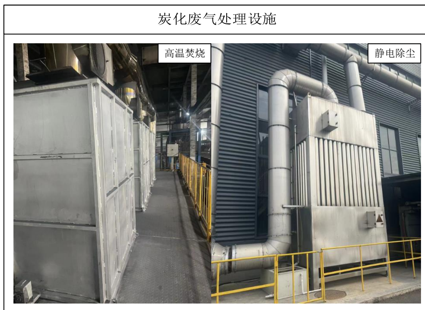
图 3-2 废气治理设施现场照片
