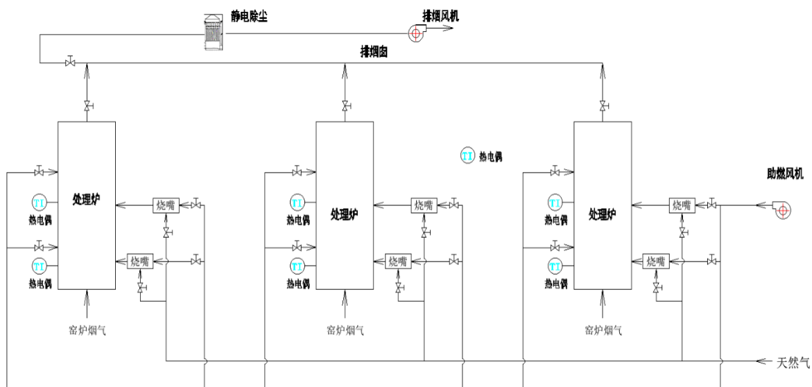
图 3-1 废气收集、治理设施示意图
