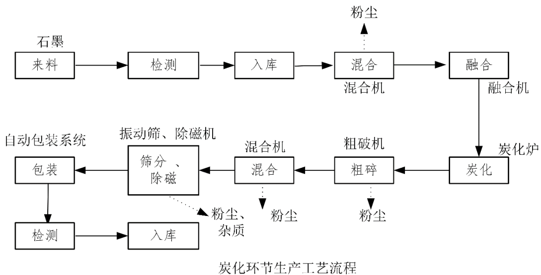
图 2-6 炭化环节工艺流程及产污环节图（环评描述）
