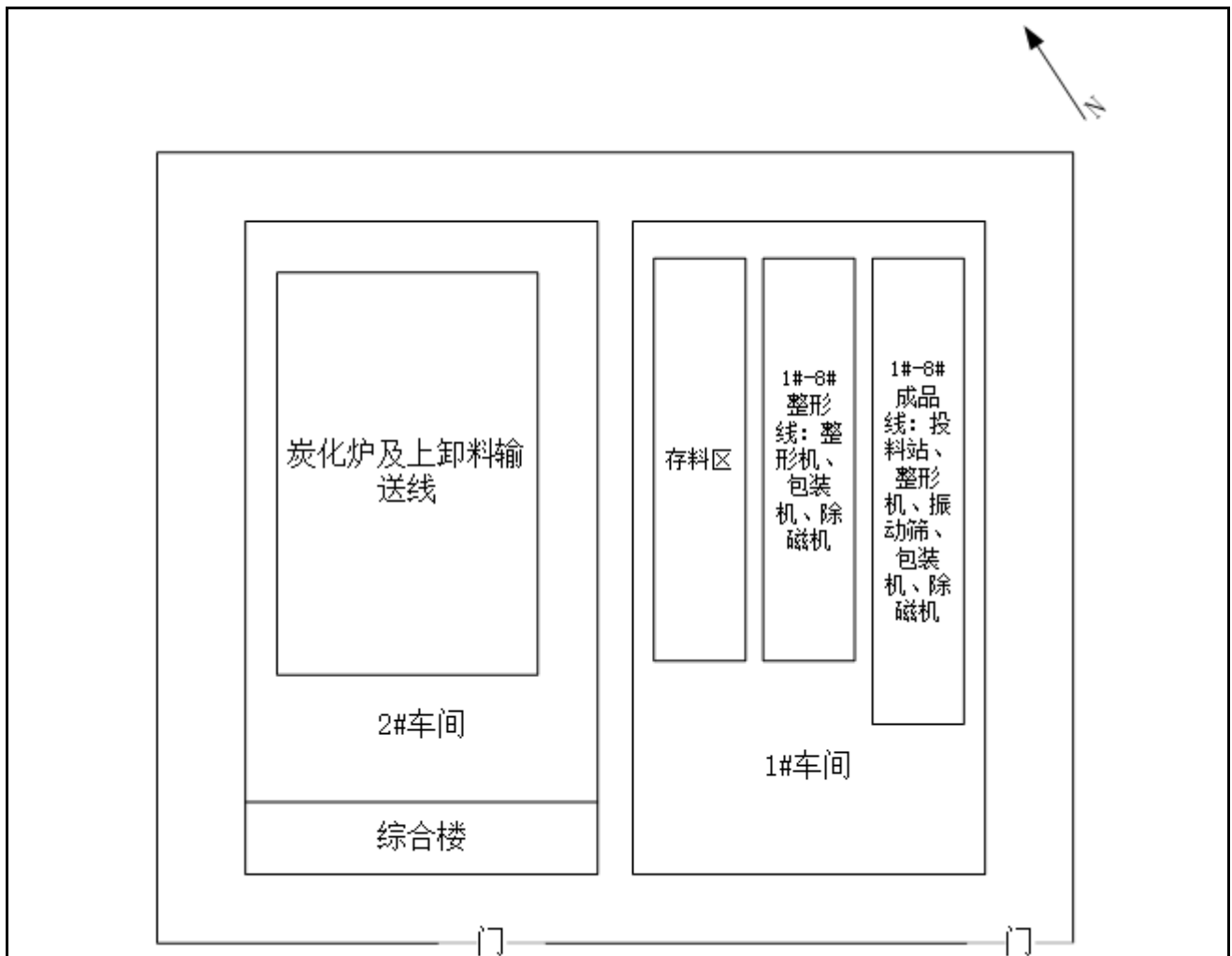
图 2-3 平面布置图
