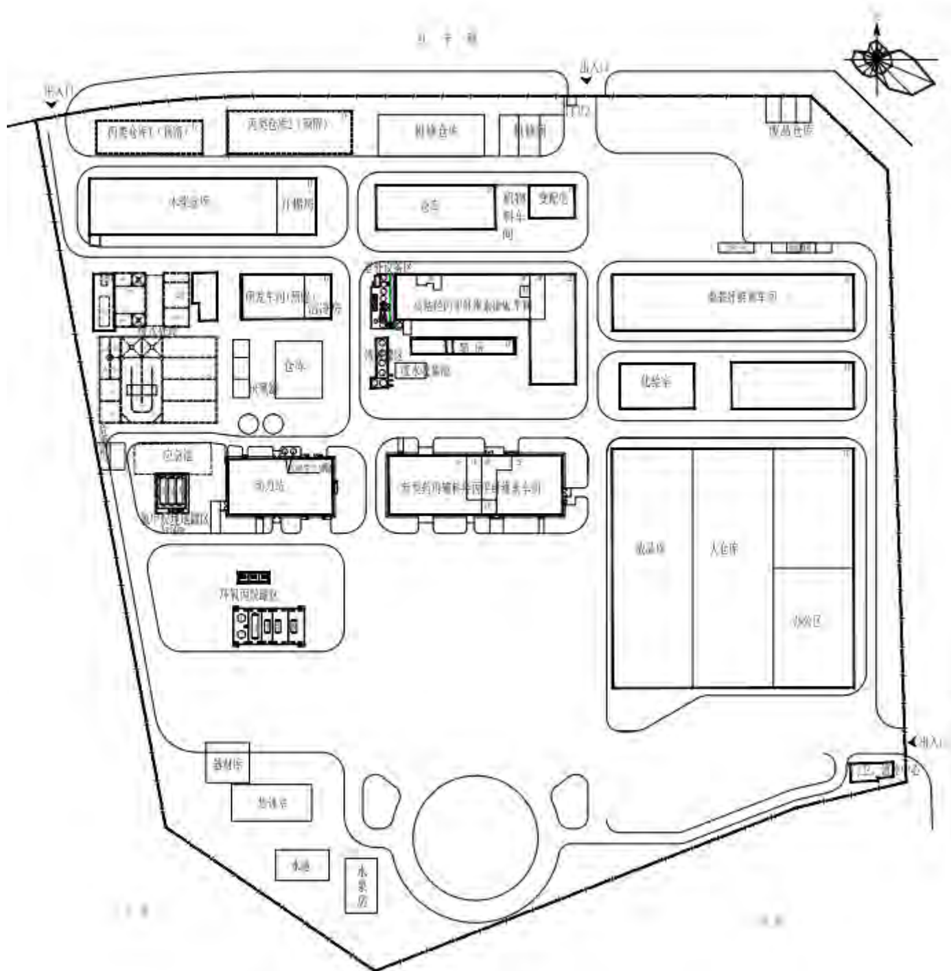
图 4.2-1 厂区总平面布置图
